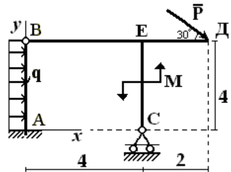
Рисунок 9 – Составная рама
