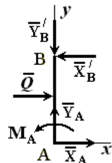
Рисунок 11 – Расчетная схема для части рамы АВ
