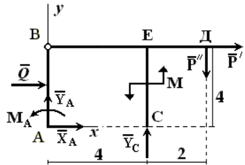
Рисунок 12 – Расчетная схема для замороженной рамы
