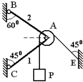
Рисунок 1. Равновесие блока
