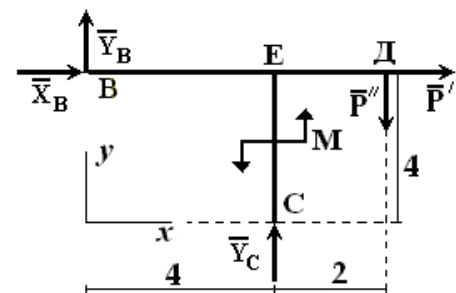
Рисунок 10 – Расчетная схема для части рамы ВСД
