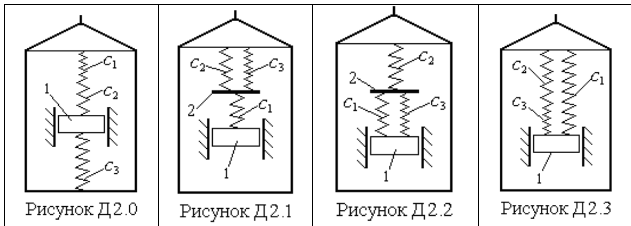
Рисунки к задачам Д2
