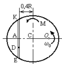
Рисунок Д 8.5а
