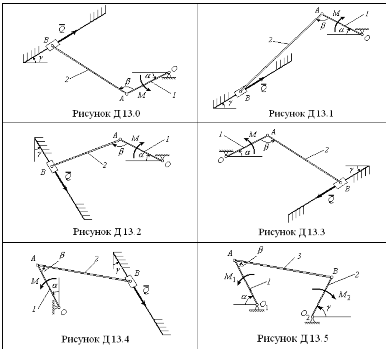
Рисунки к задачам Д13
